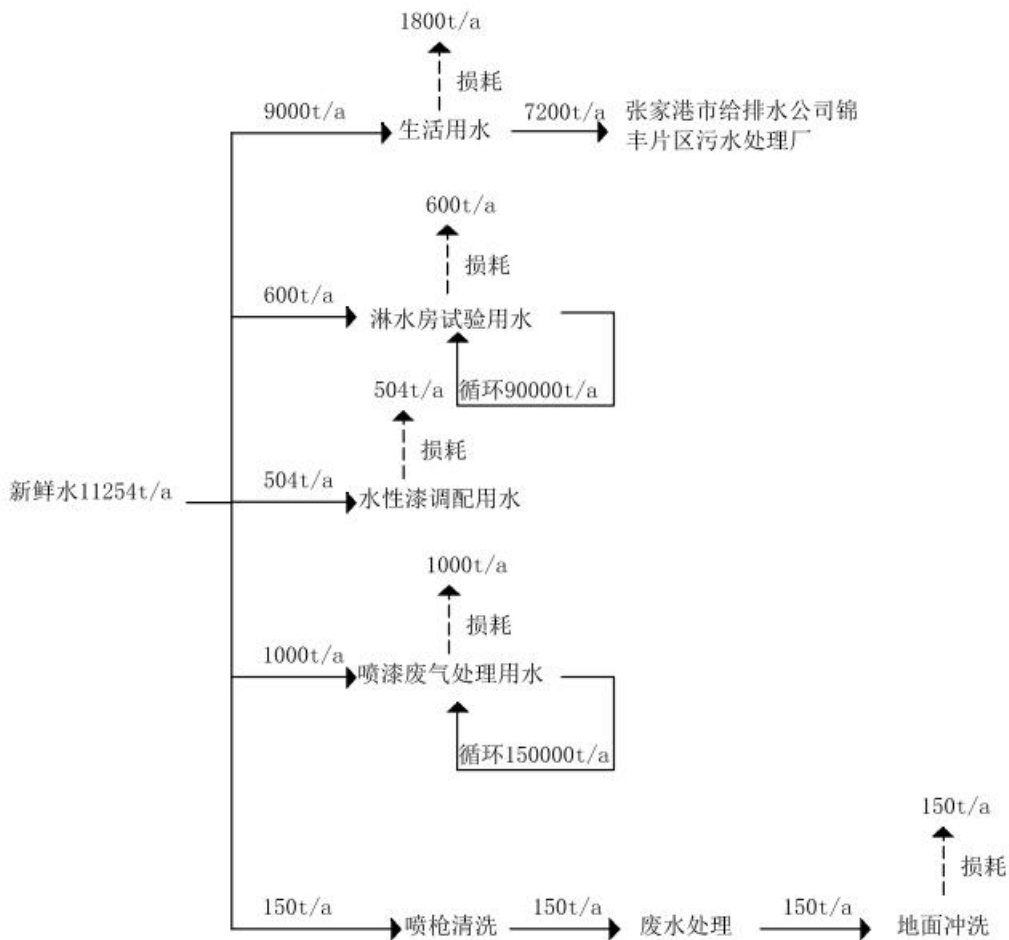
图 4.5-1 全厂水平衡图 (t/a)
