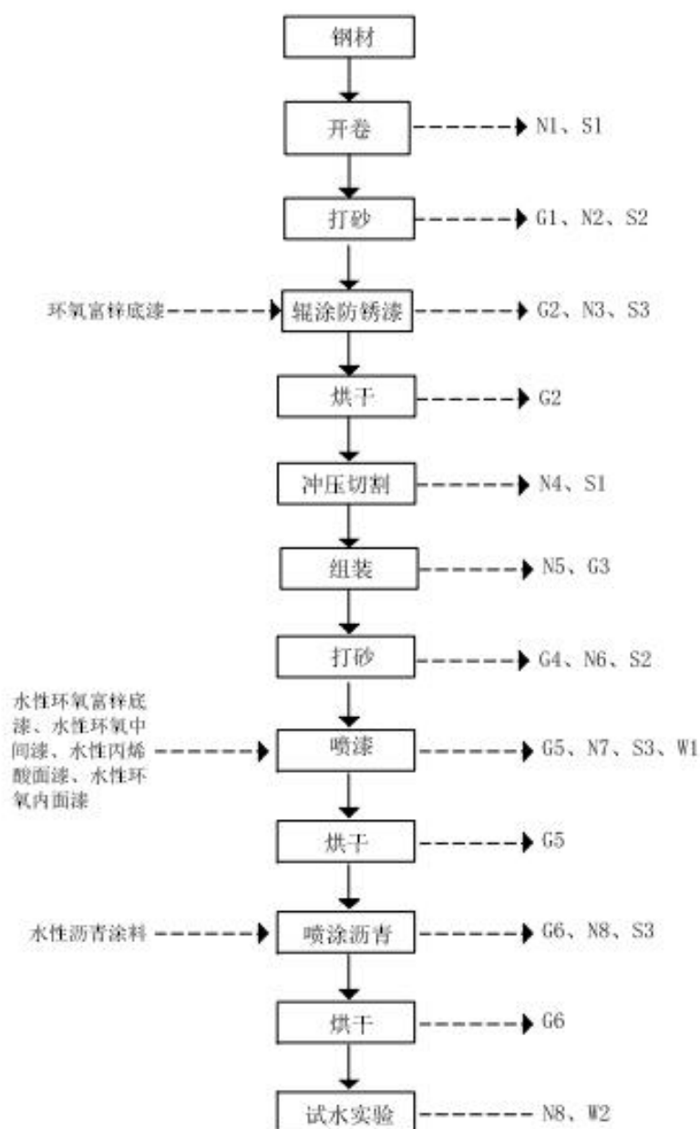
图 4.2-3 房箱配件半成品生产工艺流程图
